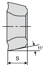
SPMX 060204-ST INOX
