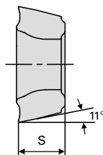
SPMX 050204-ST INOX
