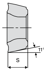
SPMX 090408-ST INOX
